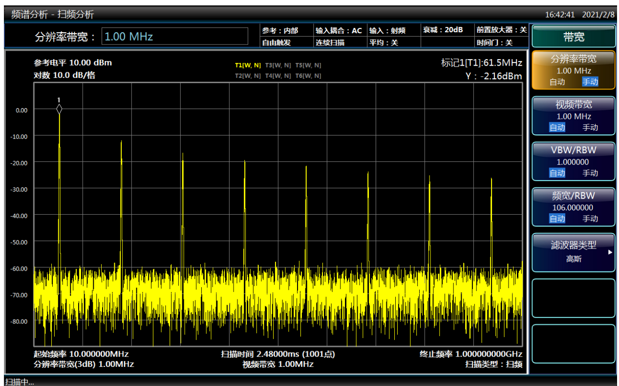
Input=0.5GHz, Pin=0dBm
